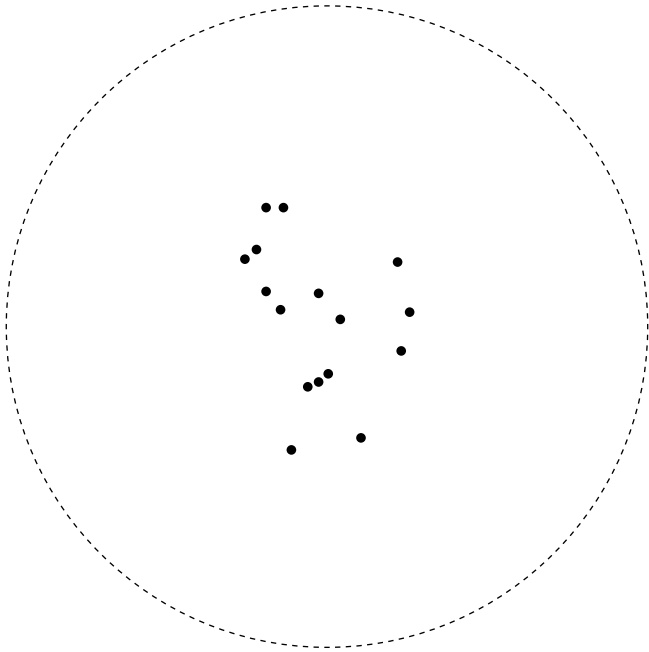
Orion
