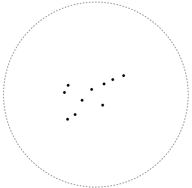
Grus
